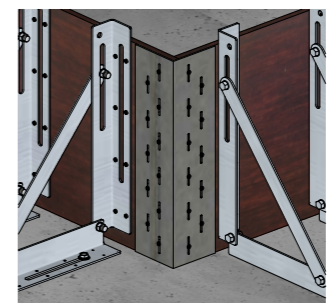
CORNER DETAIL: 1:20
